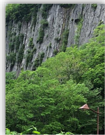
柱状節理
