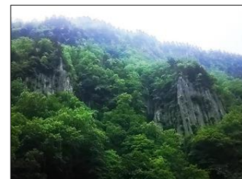
柱状节理
